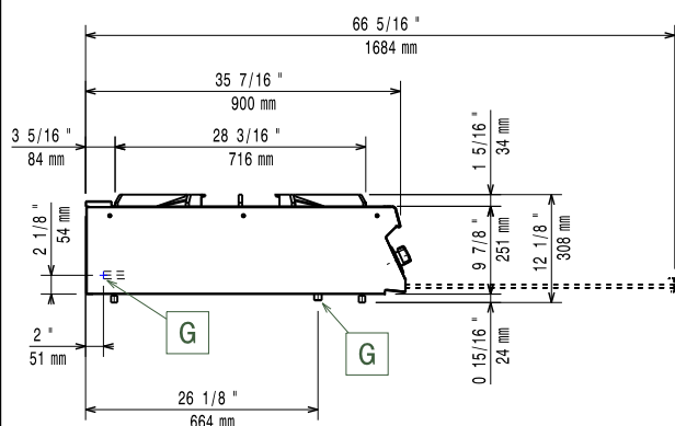
Oldalnézet
